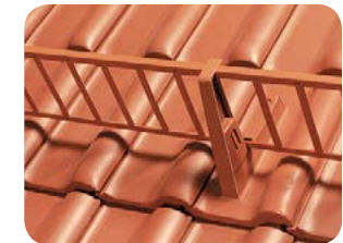
Черепица опорная с опорой под снегозадерживающую лестницу
